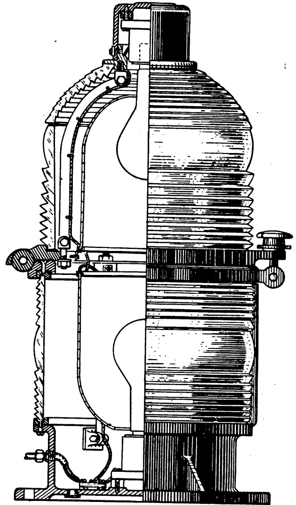
300 mm BEACON (Fresnel Lens)
