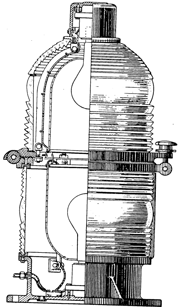
300 mm BEACON (Fresnel Lens)
